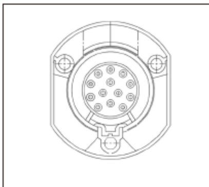
Схема определения контактов электрического разъема заднего прицепа:
